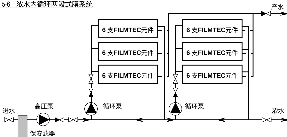
图 5-6 浓水内循环两段式膜系统
