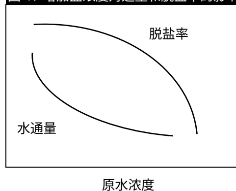
图 4. 增加盐浓度对通量和脱盐率的影响
