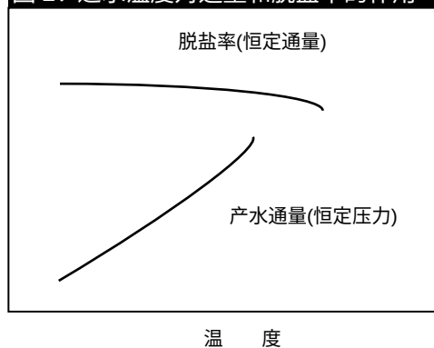
图 2. 进水温度对通量和脱盐率的作用
