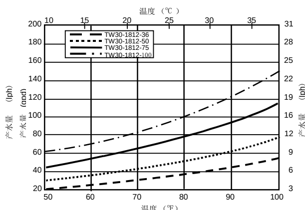
温度对产水量的影响 (恒定压力和回收率)
