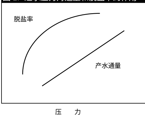
图 1. 进水压力对通量和脱盐率的作用
