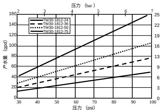
压力对产水量的影响 (恒定温度和回收率)
