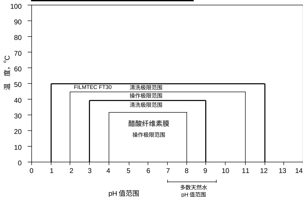
图 3. FT30 超薄复合膜和 CA 膜运行和清洗参数比较
