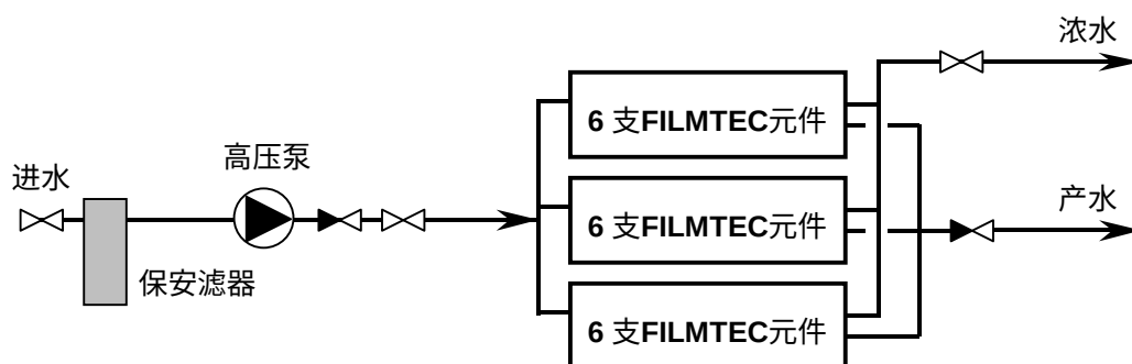
图 5-4 单段系统
