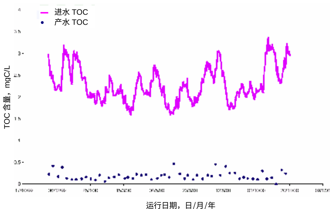
图 12 进水和产水 TOC 含量 (mgC/L)
