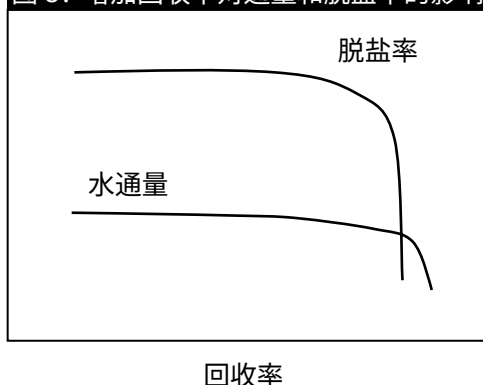
图 5. 增加回收率对通量和脱盐率的影响
