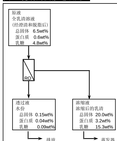
图 3 乳清的反渗透法处理
