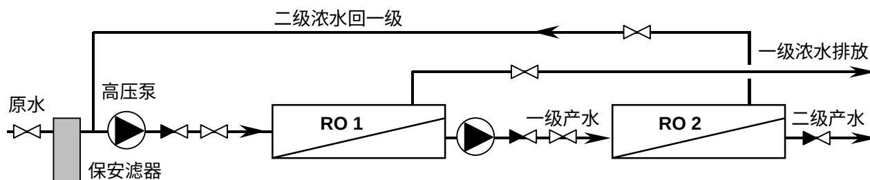
图 5-9 二级反渗透系统
