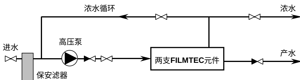
图 5-3 单组件系统
