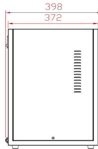
左侧视图
