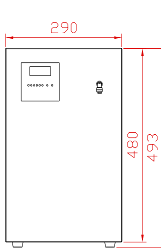
正面视图
