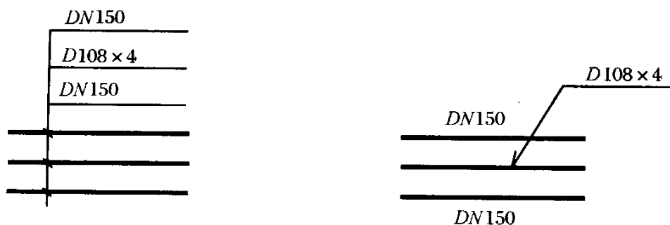
图 2.4.3-2 多管管径表示法
