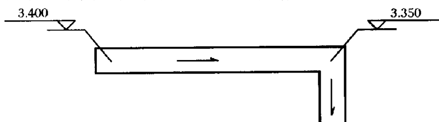
图 2.3.5-2 平面图中沟渠标高标注法
