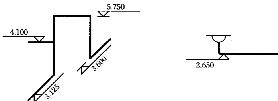
图 2.3.5-4 轴测图中管道标高标注法
