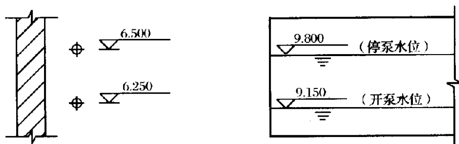
图 2.3.5-3 剖面图中管道及水位标高标注法
