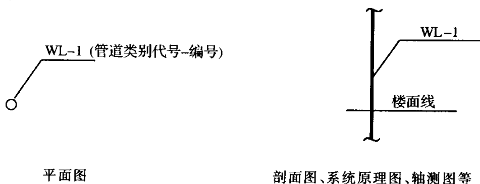
图 2.5.2 立管编号表示法
