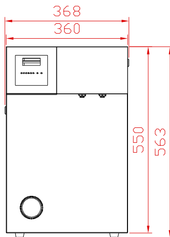
正面视图
