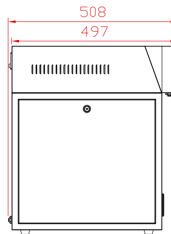
左侧视图
