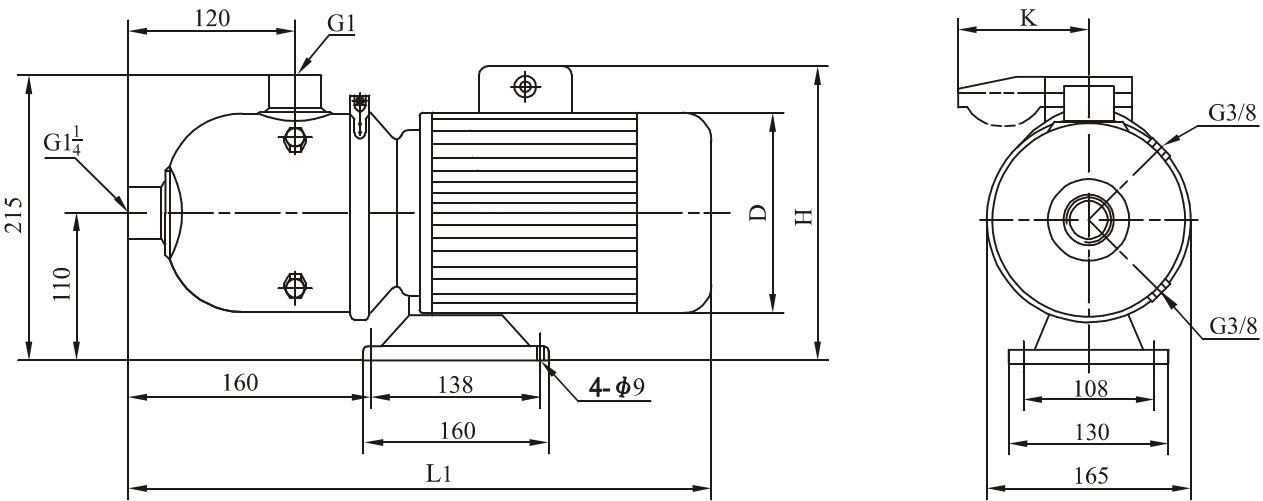
安装图
