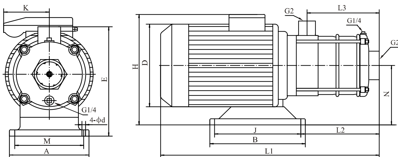
尺寸和重量
