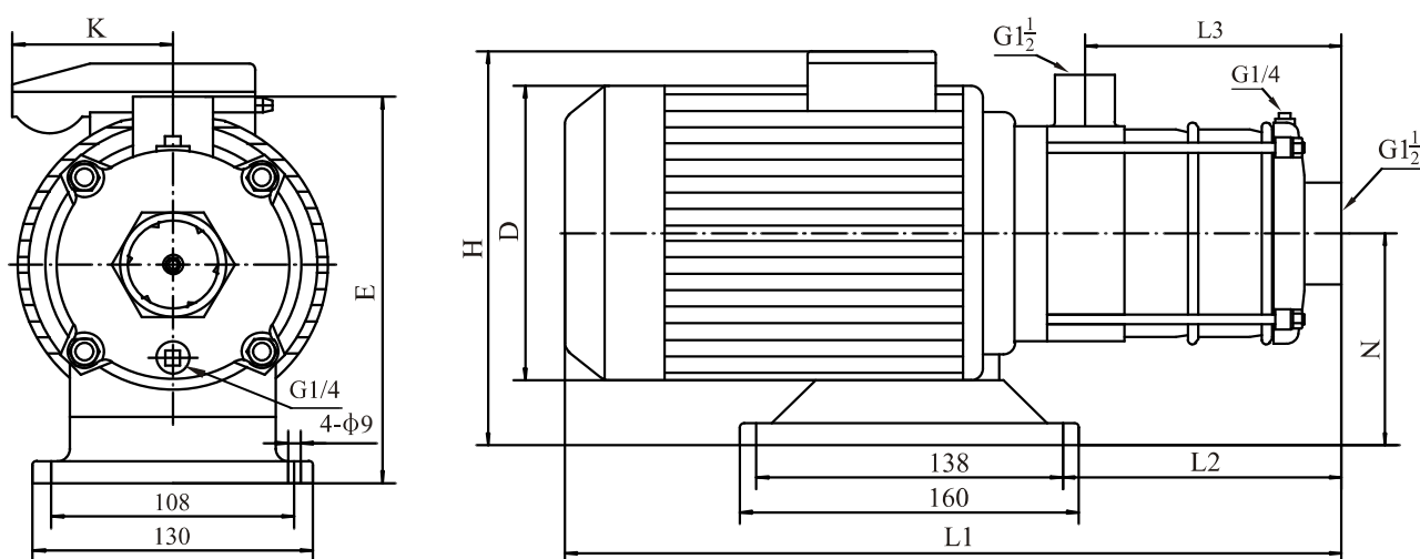
尺寸和重量
