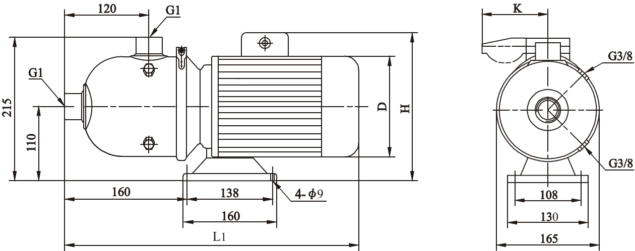
安装图
