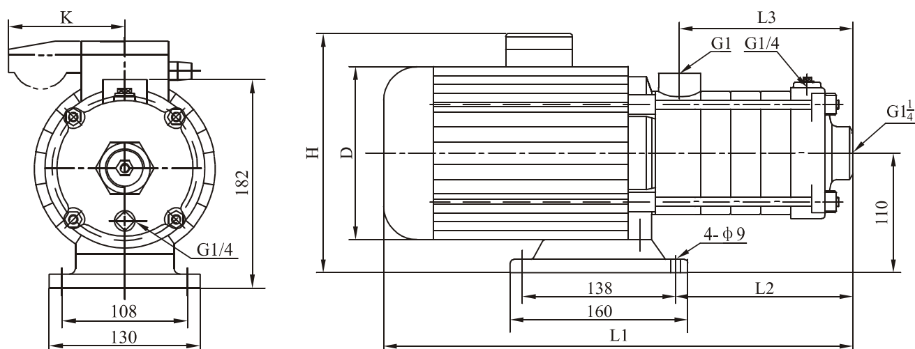
尺寸和重量
