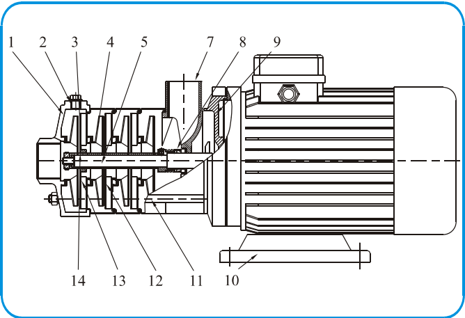
截面图 CHLF,CHLF(T)
